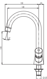
Pipa samozapiralna umivalnik Slavina samozatvarajuća umivaonik Self closing basin tap
