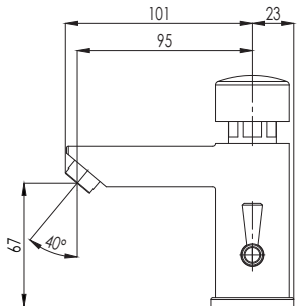
Armatura samozapiralna umivalnik Slavina samozatvarajuća umivaonik Self closing basin mixer
